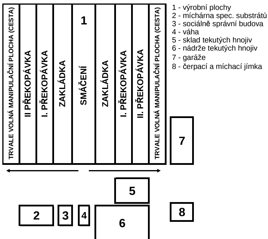
Obr. 22.2: Pohyb kompostovacích hromad a vybavení kompostárny při aplikaci tekutých hnojiv
